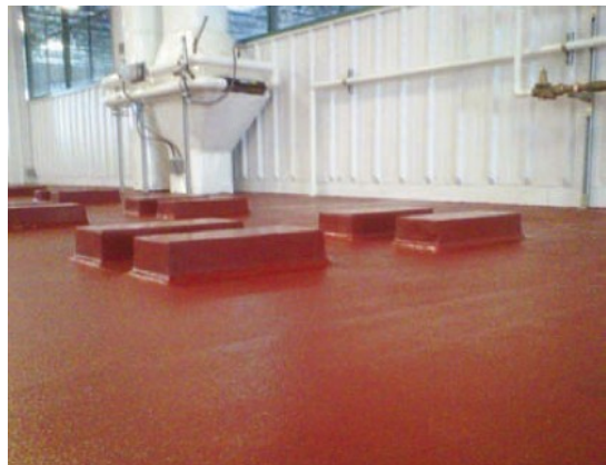
Stonhard在Shearer's 俄亥俄州马西隆市的生产厂房使用了Stonclad UT 砂浆和Stonset TG6 薄浆做的设备支脚垫板。
